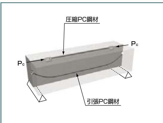
軸応力
